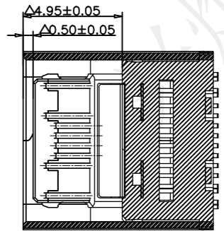
截面B-B
