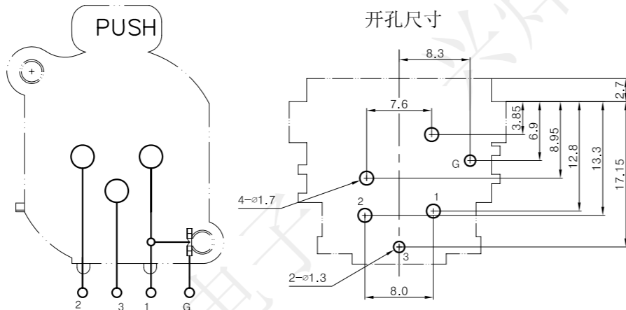
通电原理
