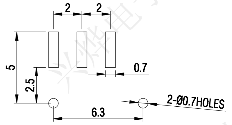
P.C.B LAYOUT DIMENSION
